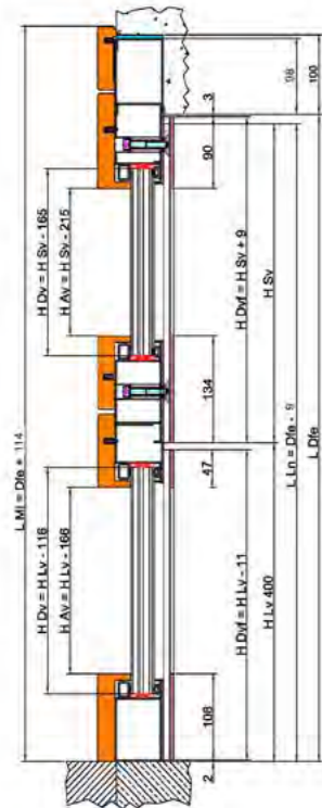
LATERALE SOPRALZO LATERAL TRANSOM
