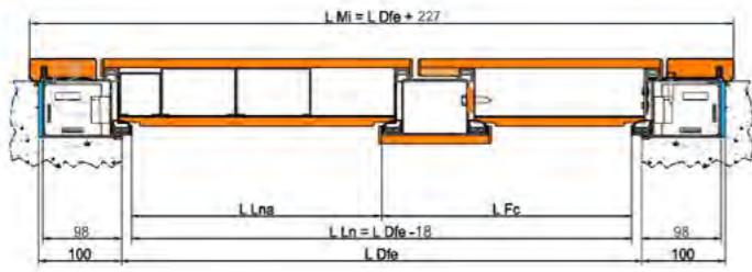
OLTRE LUCE WALL BEHIND
