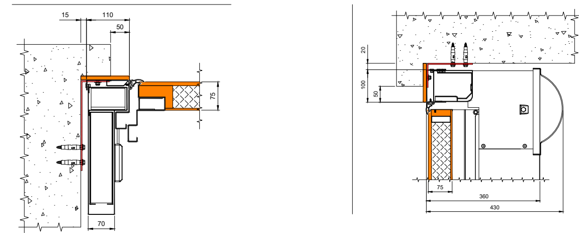
DETAGLIO TELAI0 PARZIALMENTE IN LUCE SEZIONE ORIZZONTALE DÉTAIL DU CADRE PARTIELLEMENT EN TABLEAU COUPE HORIZONTALE
