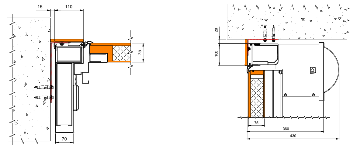
DETAGLIO TELAI0 IN LUCE SEZIONE ORIZZONTALE SECTION HORIZONTALE
